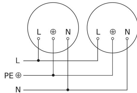
Schéma du circuit d'interconnexion maître/esclave
